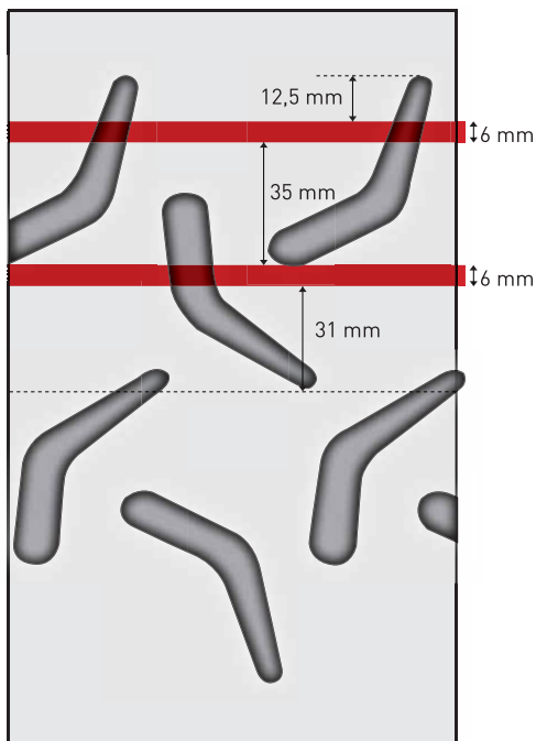
DIMENSIONS & TYPE DU PNEUMATIQUE 200/615-17 C03 Pneu du Rallye Asphalte Moulé
