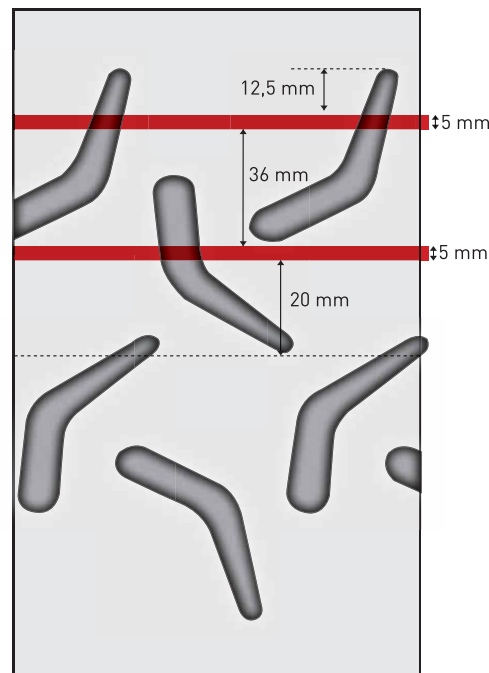
DIMENSIONS & TYPE DU PNEUMATIQUE 170/600-16 C03 Pneu du Rallye Asphalte Moulé
