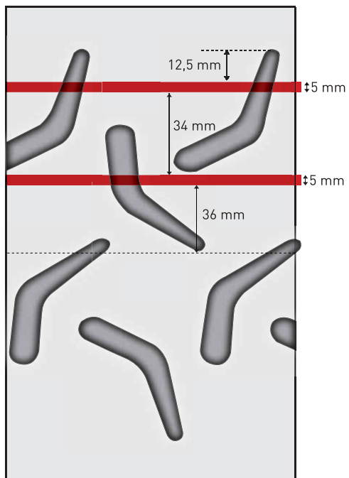
DIMENSIONS & TYPE DU PNEUMATIQUE 220/580-15 C03 Pneu du Rallye Asphalte Moulé
