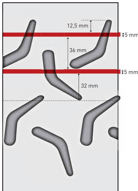
DIMENSIONS & TYPE DU PNEUMATIQUE 200/580-15 C03 Pneu du Rallye Asphalte Moulé
